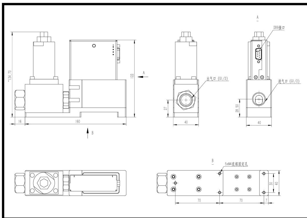
量程 200SLPM 负压使用尺寸图
