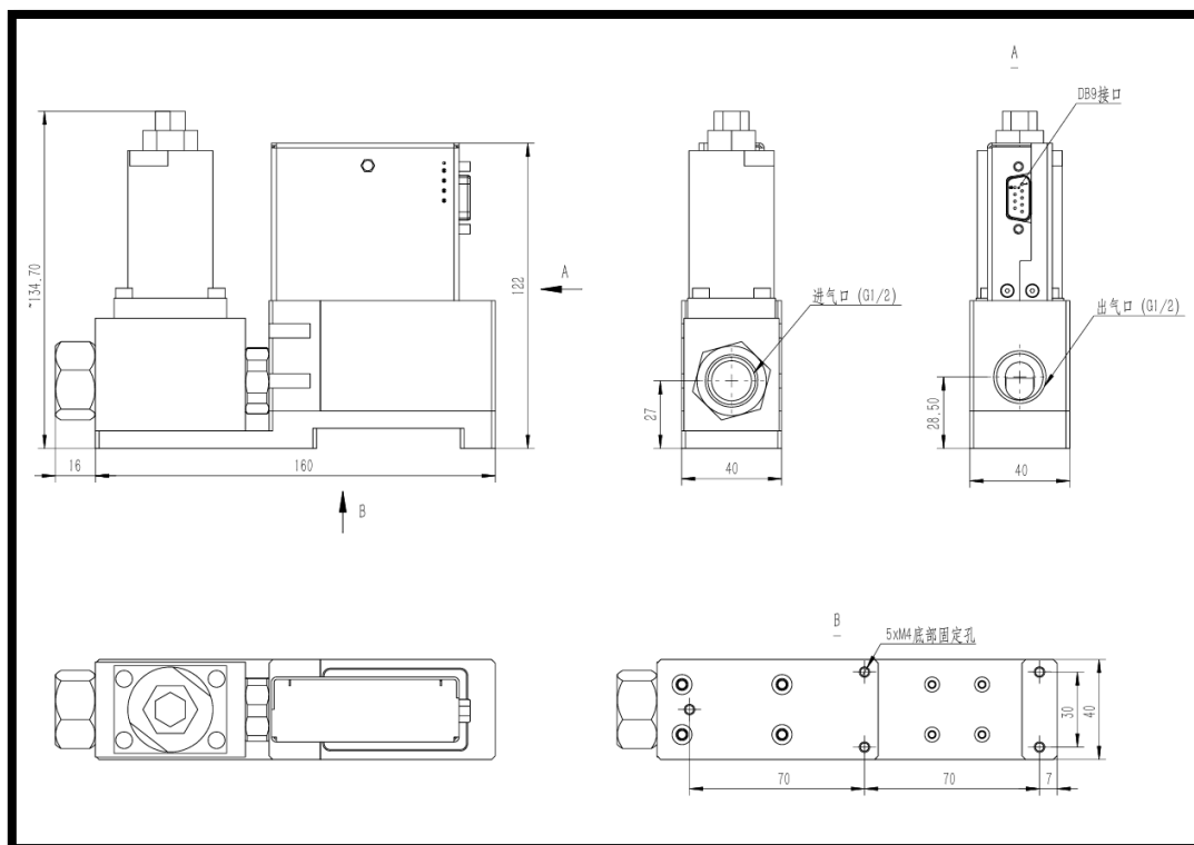
量程 200SLPM 正压使用 GF03 尺寸图
