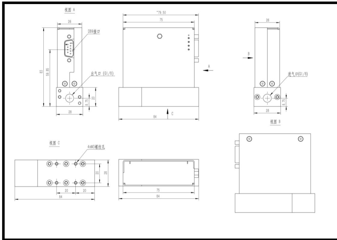
量程 200SCCM-10SLPM 正压使用 GF03 尺寸图
