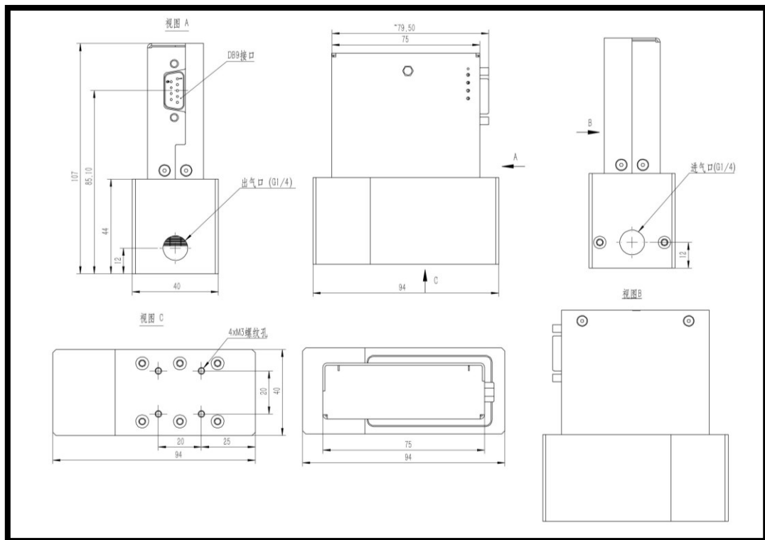
量程 50SSLPM-100SLPM 正压使用 GF03 尺寸图
