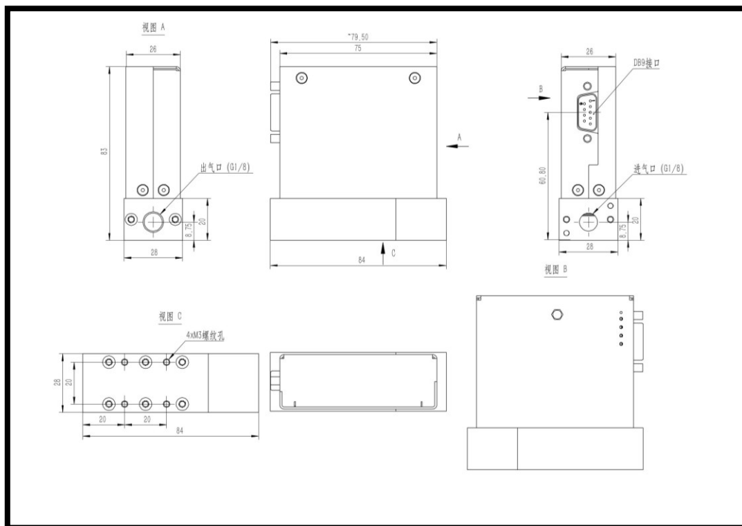
量程 200SCCM-10SLPM 负压使用 GF03 尺寸图
