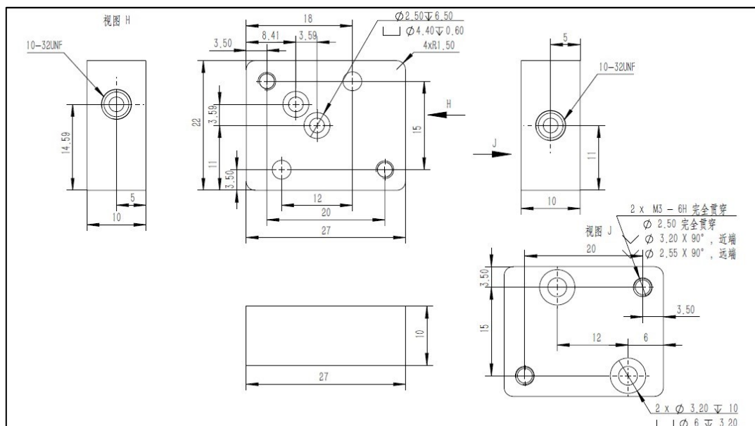
GT200 减压型\GT201 背压型底座尺寸
