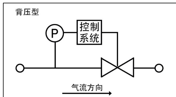
GT201 背压型压力控制器
