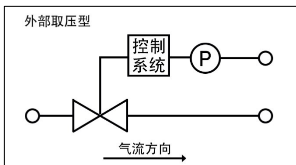
GT202 外部取压型压力控制器
