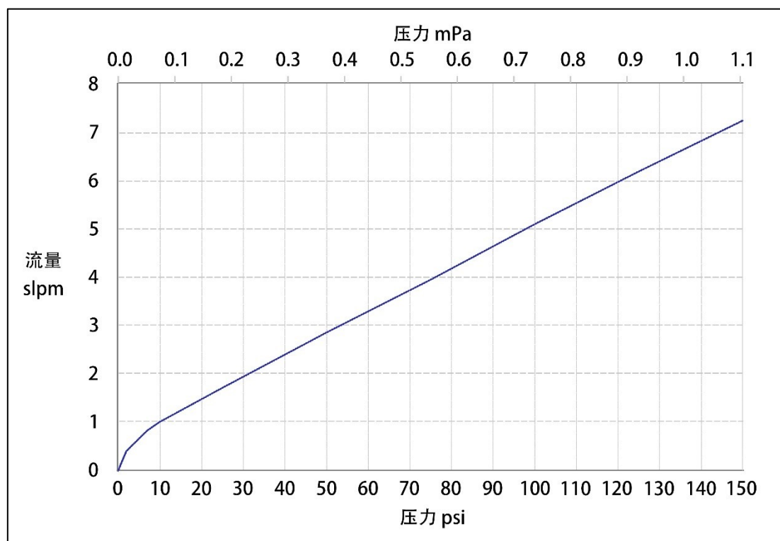
型号 2 气体流量通过性曲线
