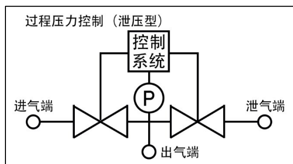
GT203 过程控制型（泄压型）压力控制器
