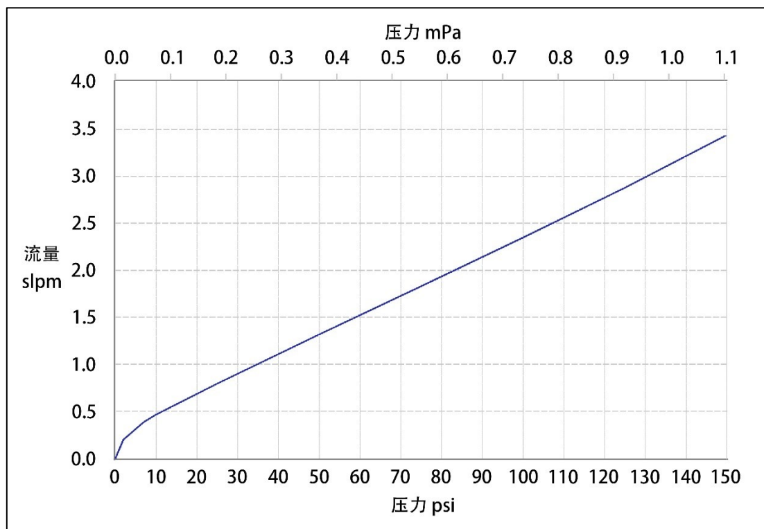
型号 1 气体流量通过性曲线
