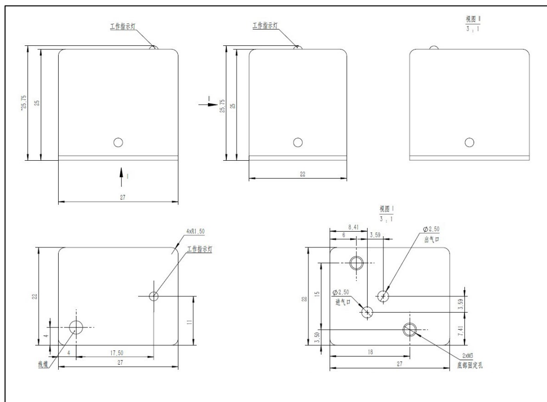
GT200 减压型\GT201 背压型无底座尺寸图
