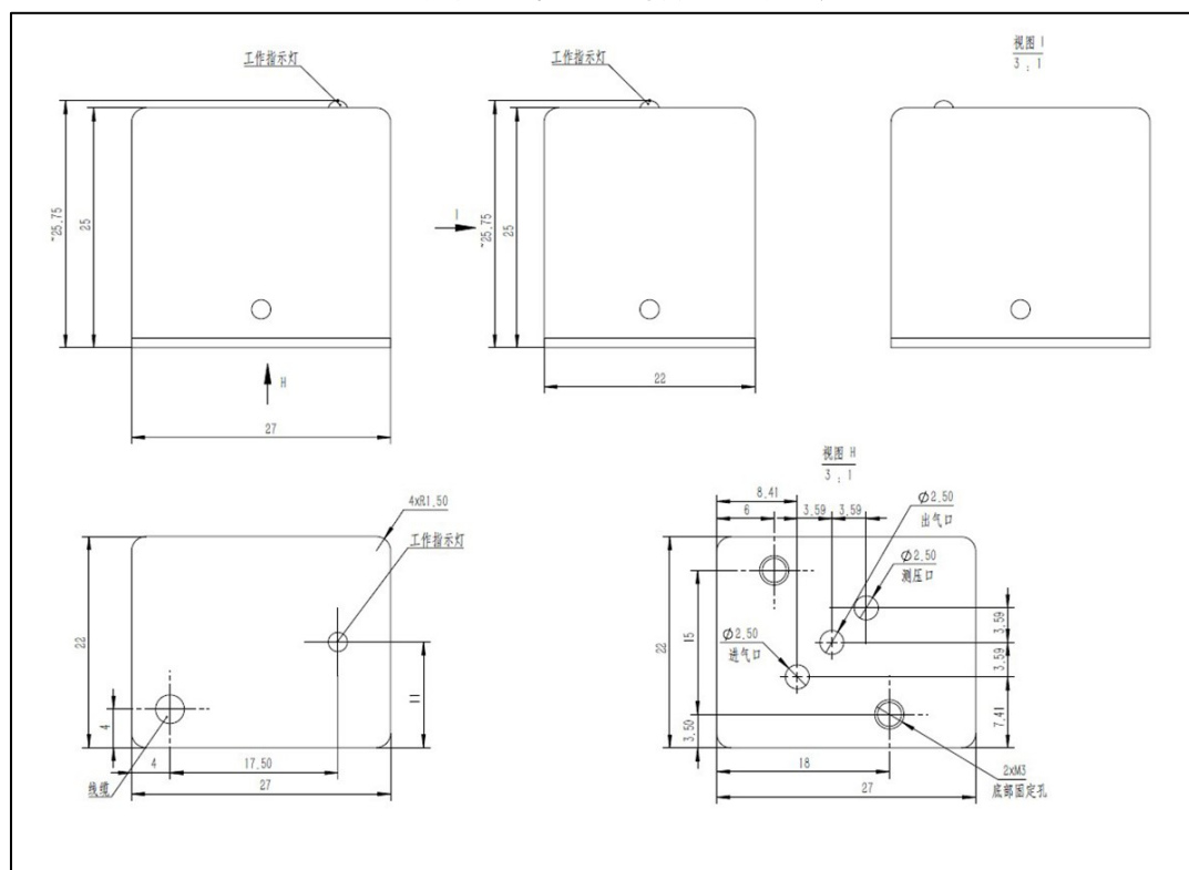
GT202 外部取压型产品尺寸图
