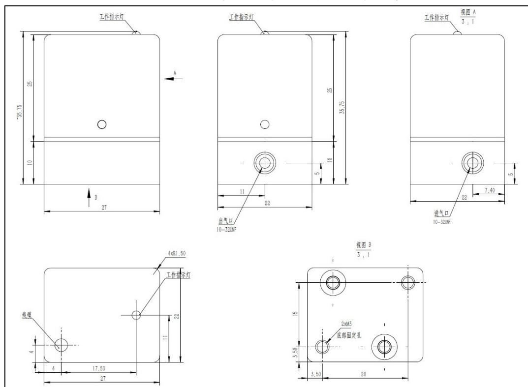
GT200 减压型\GT201 背压型含底座尺寸图
