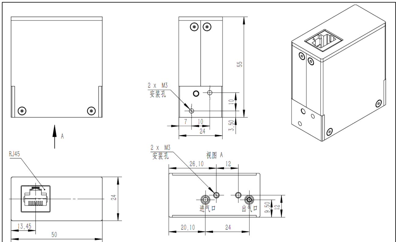
GT230 尺寸图
